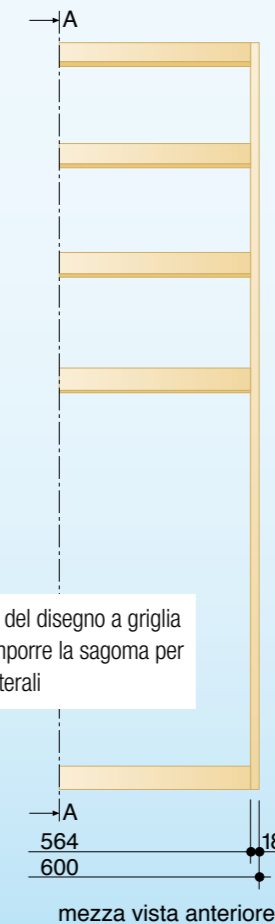
4 Nei listellari creare due fori ciechi per parte. Gli sciabloni per tasselli aiutano a segnare le misure
