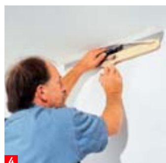
4 Tagliare anche i pezzi in eccesso del tessuto trend con una lamiera da taglio ed il taglierino
