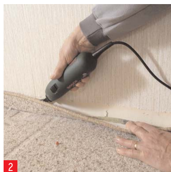
2 Con un'avvitatrice manuale o elettrica togliere dapprima il battiscopa del tappeto e poi il tappeto.
