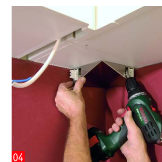
04 Fissate il modulo angolare al quale devono essere fissati i singoli moduli.
