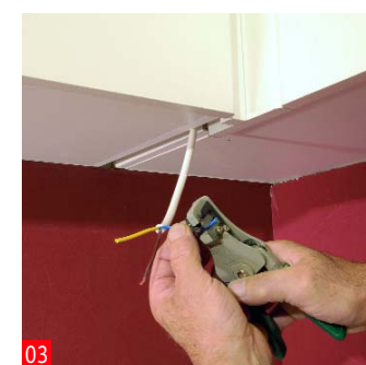
03 Ora preparate i cavi in modo da poterli collegare al modulo dell'interruttore.
