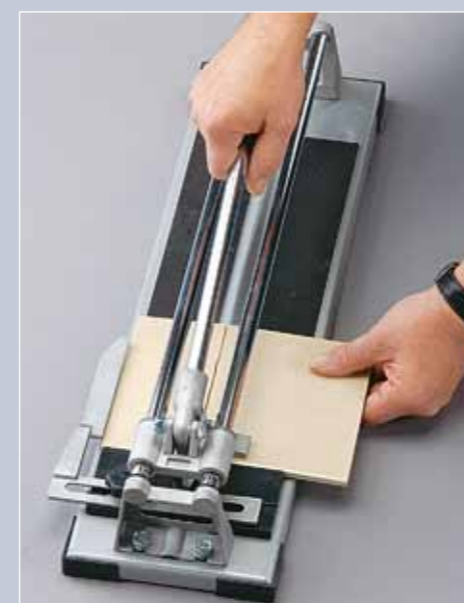
La piastrella si spezza lungo la linea scalfita. Segno di qualità: la battuta d'arresto regolabile.
